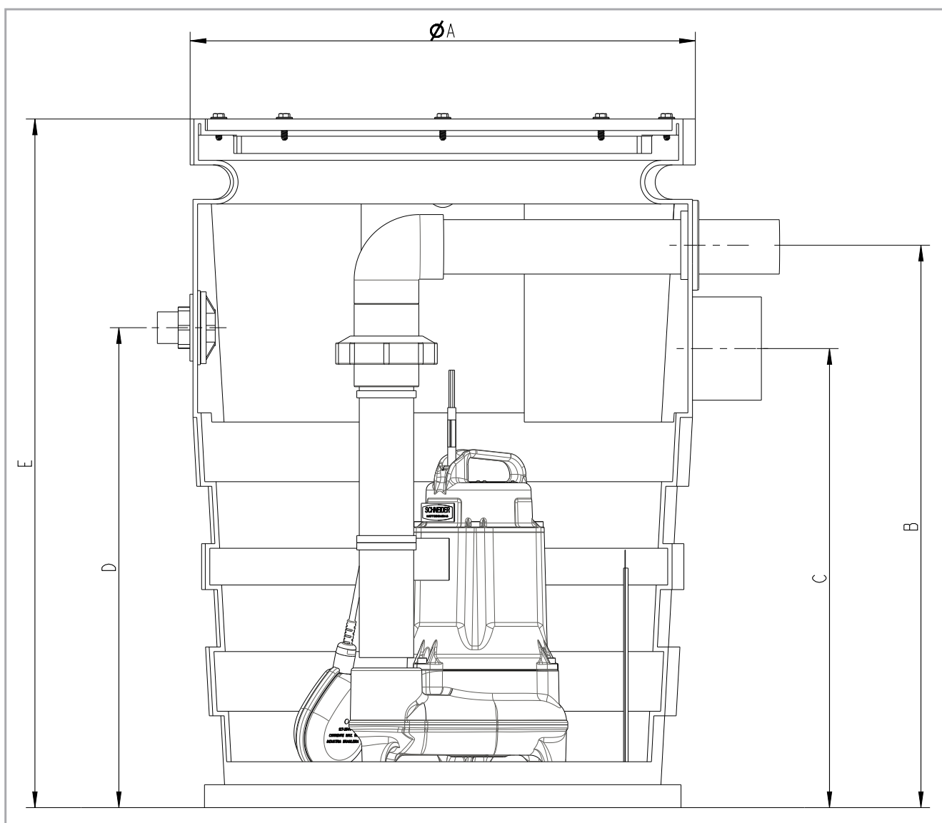
Dimensões em Milímetros (mm)
